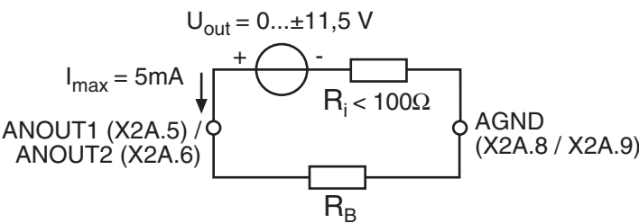
Fig. 7.2.10 Analog output
